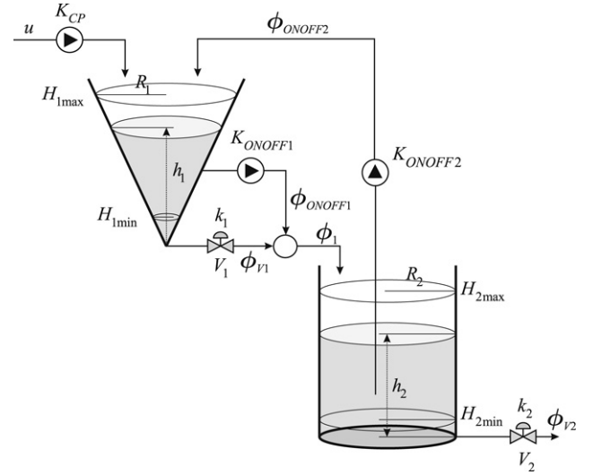
Fig. 4. The tank-system plant.
